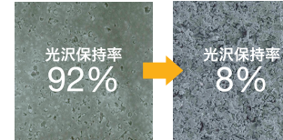
塗膜表面を電子顕微鏡で5000倍に拡大して撮影
