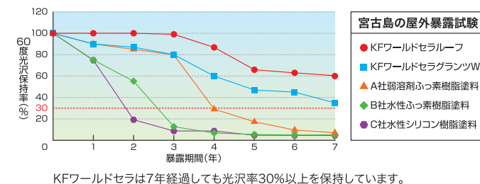
KFワールドセラは7年経過しても光沢率30%以上を保持しています。
